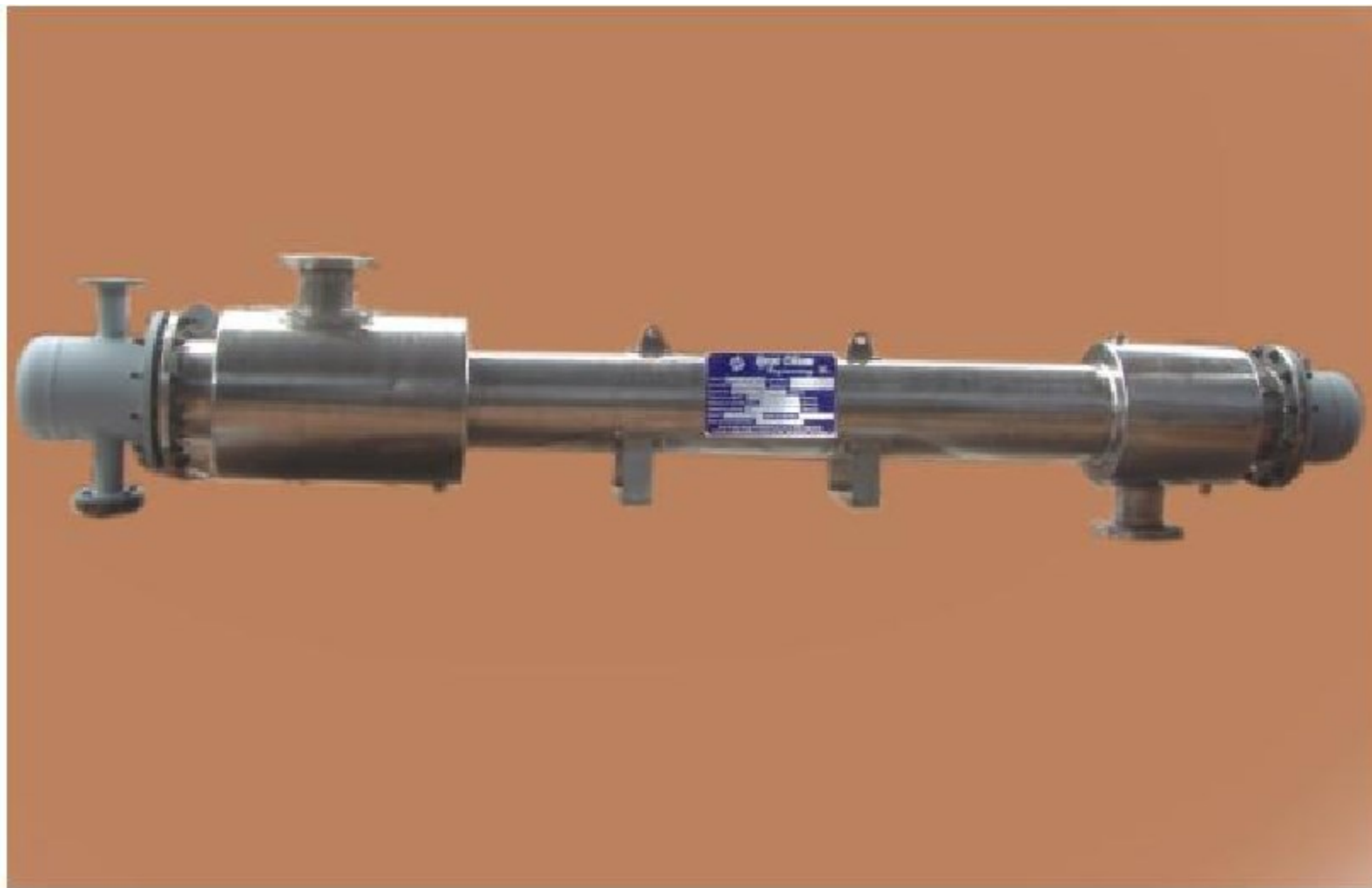
CO2 Gas Cooler s.s .
